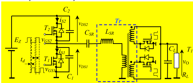
Rezonansowa przetwornica napięcia typu LLC (36-60V//12V/60W, sprawność maksymalna 92%)
