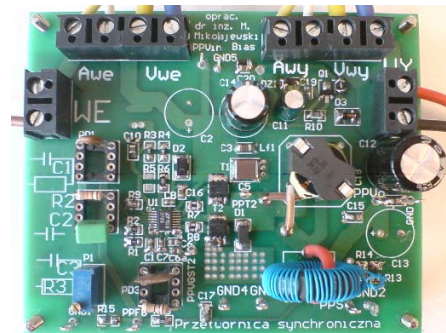
Synchroniczna przetwornica obniżająca V_{we}=15-30V, V_{wy}=12V/5A
