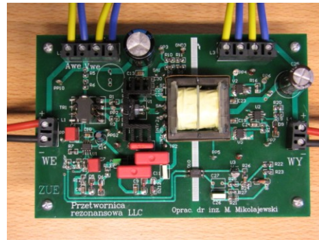
Rezonansowa przetwornica napięcia typu LLC (36-60V//12V/60W, sprawność maksymalna 92%)
